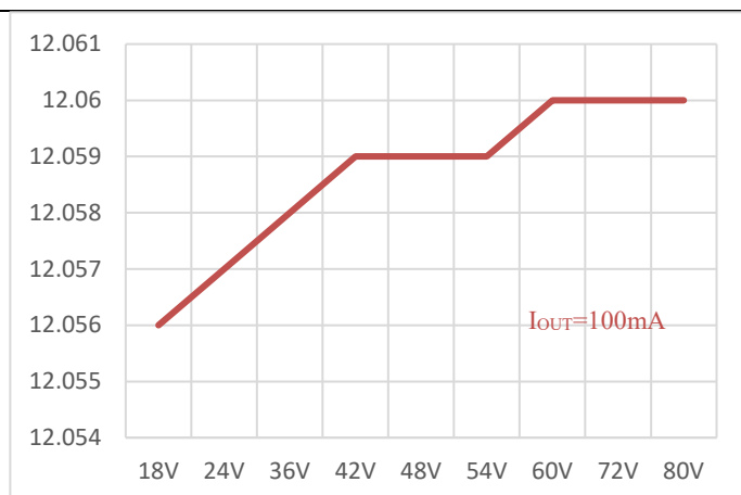
图2 线性调整
