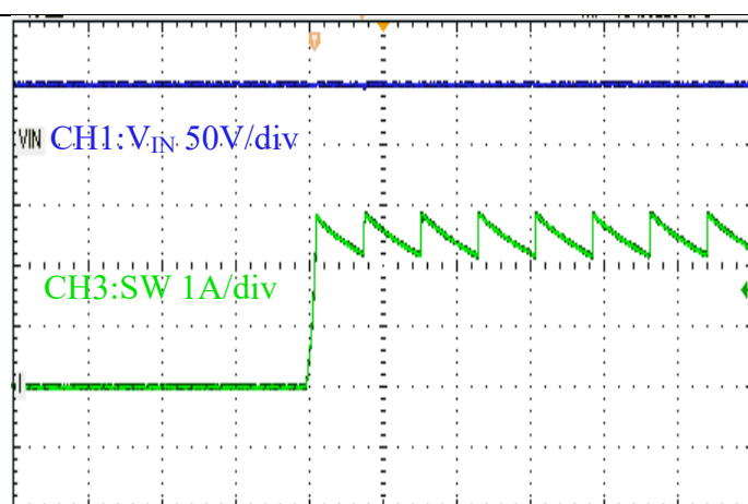
图 10 上电带载 1A 短路
