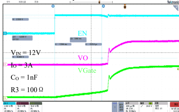
EN turnon external MOSFET
