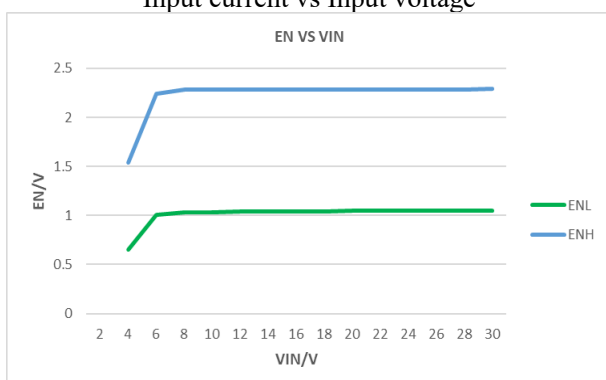
EN vs Input voltage
