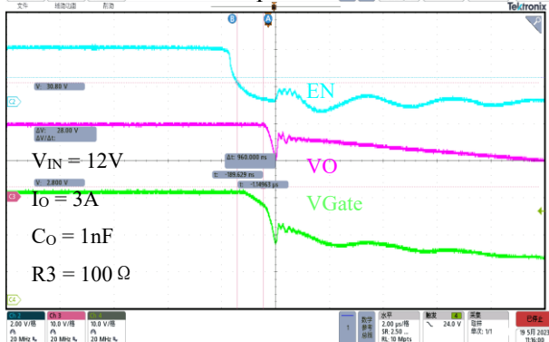
EN turnoff external MOSFET
